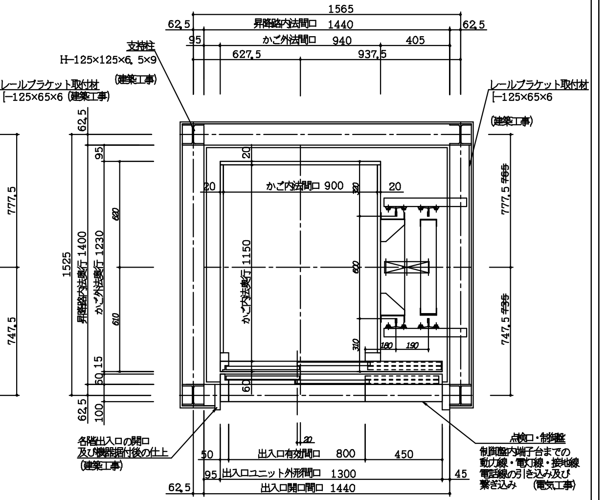
2階 昇降路平面図
