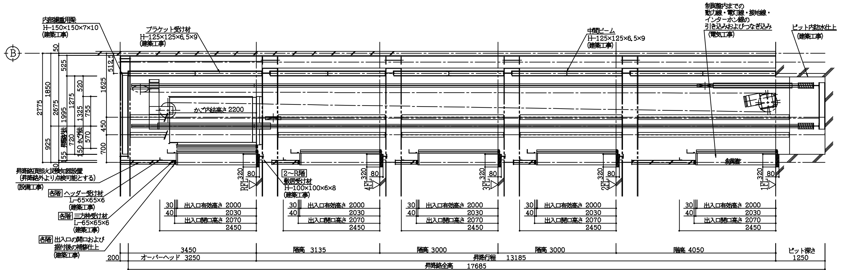
昇降路断面図 S=1/40
